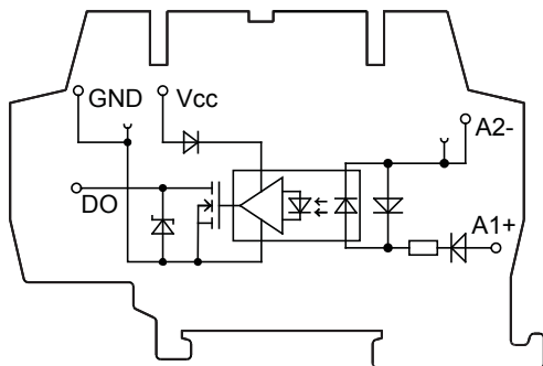
Рис. 4.1 Функциональная схема твердотельного реле
