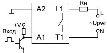
г) нормально закрытый контакт реле, управление NPN транзистором
