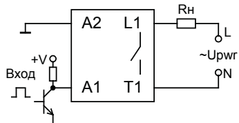
г) нормально закрытый контакт реле, управление NPN транзистором
